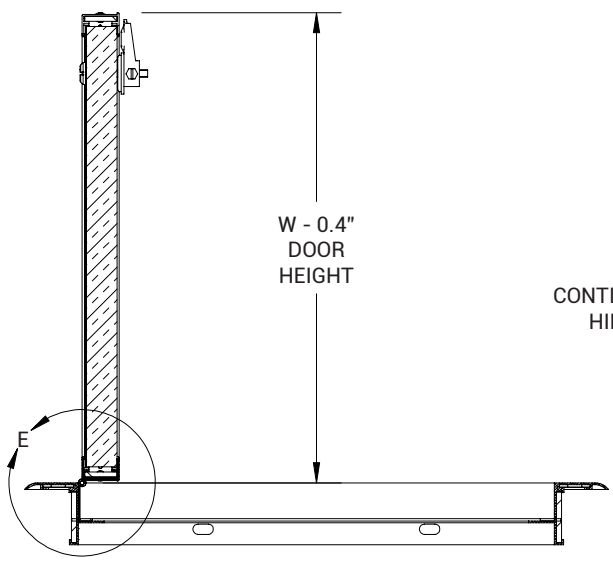
SECTION D-D
