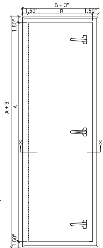
ELEVATION
