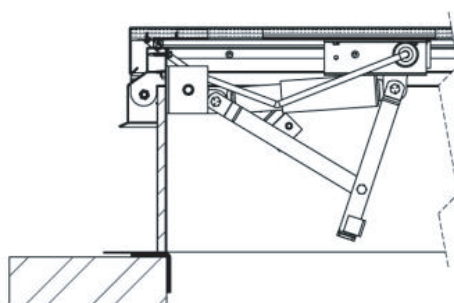
RSGD Drop-In
