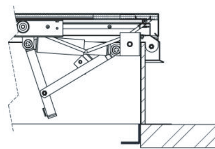
RSGB Bolt-In
